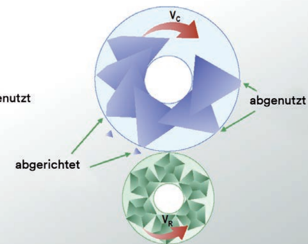
Abrichtverhalten mit 3M™ Precision-Shaped Grain
