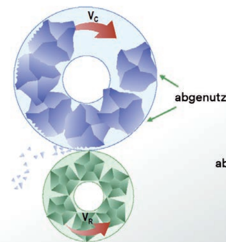
Abrichtverhalten Standard-Sinterkorund
